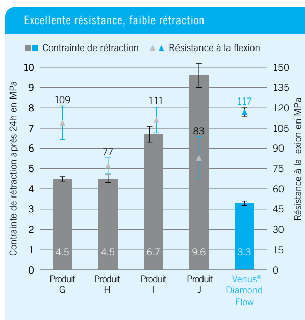
Source: R&D de Kulzer, Wehrheim, Allemagne. Non publié. Données fichées.
